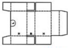
Modelo ABNT 0444
